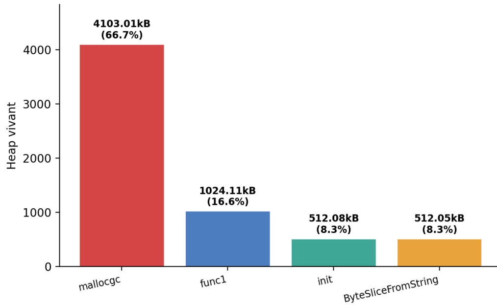
Figure — Heap Go encore vivant par fonction (pprof -inuse_space).
