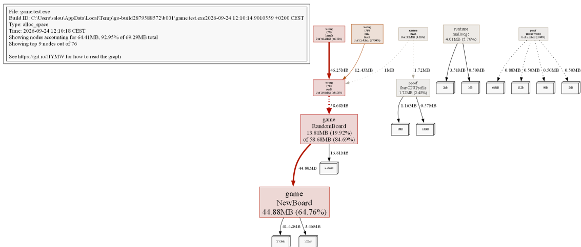
Figure — Graphe d'appels mémoire (go tool pprof -png).
