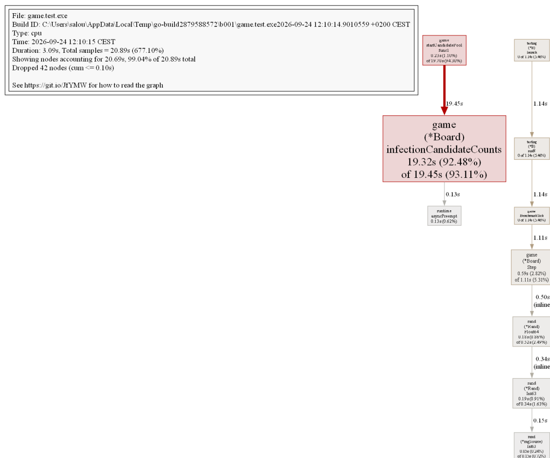
Figure — Graphe d'appels CPU (go tool pprof -png).
